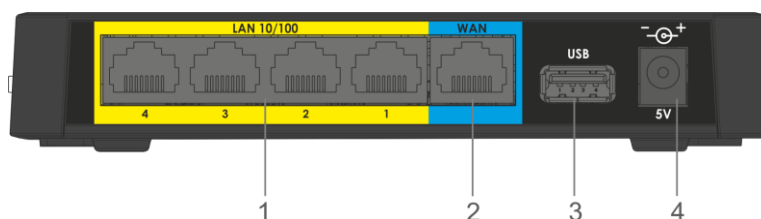
Рисунок 3 – Внешний вид задней панели RG-35-Wac
