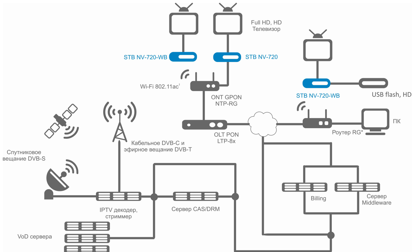
Рисунок 1 – Схема применения
