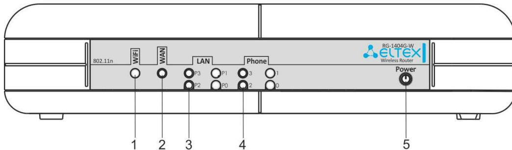
Рисунок 5 – Внешний вид передней панели RG-1404G-W.
