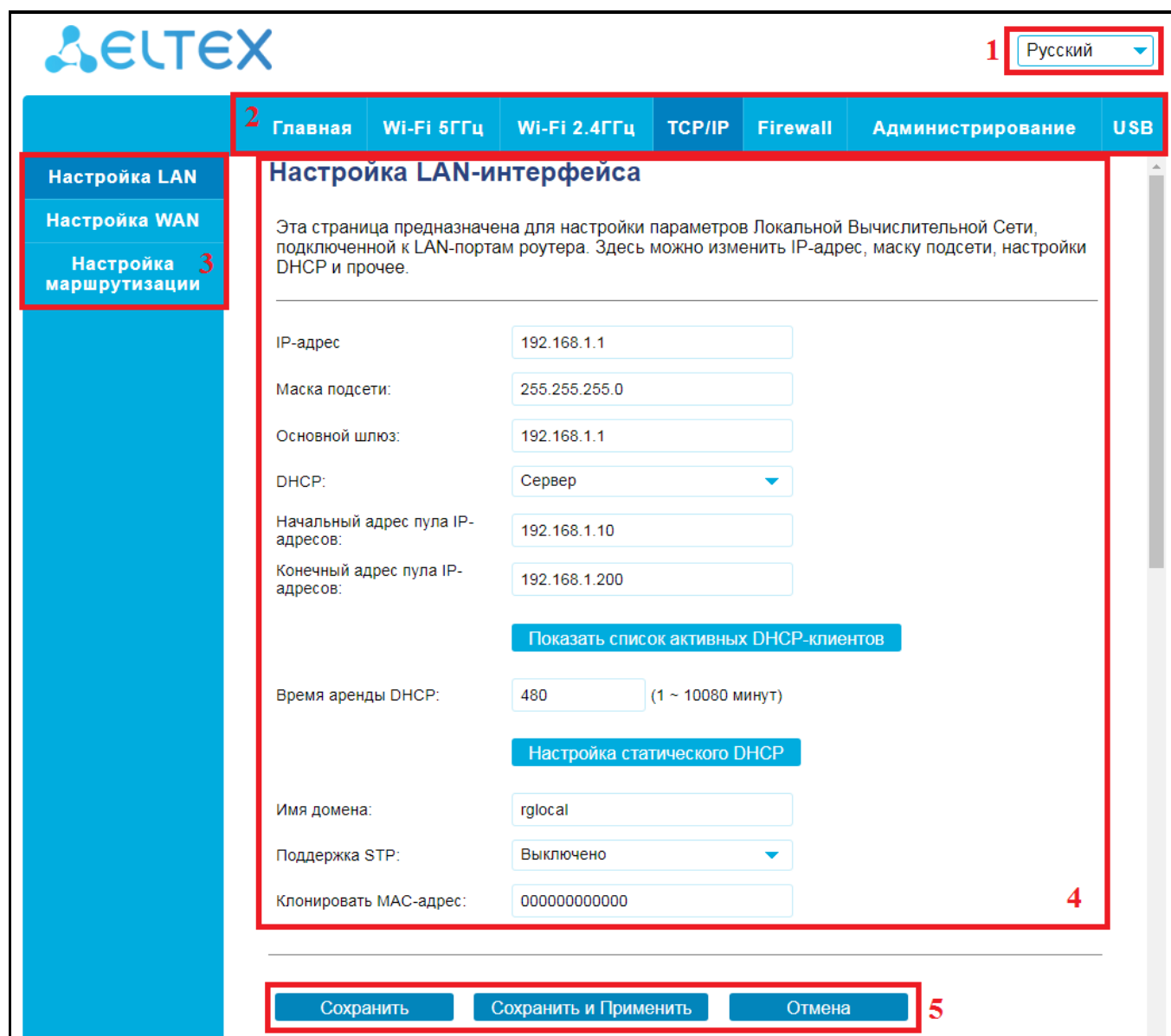
Рисунок 5 — Элементы навигации web-конфигуратора
