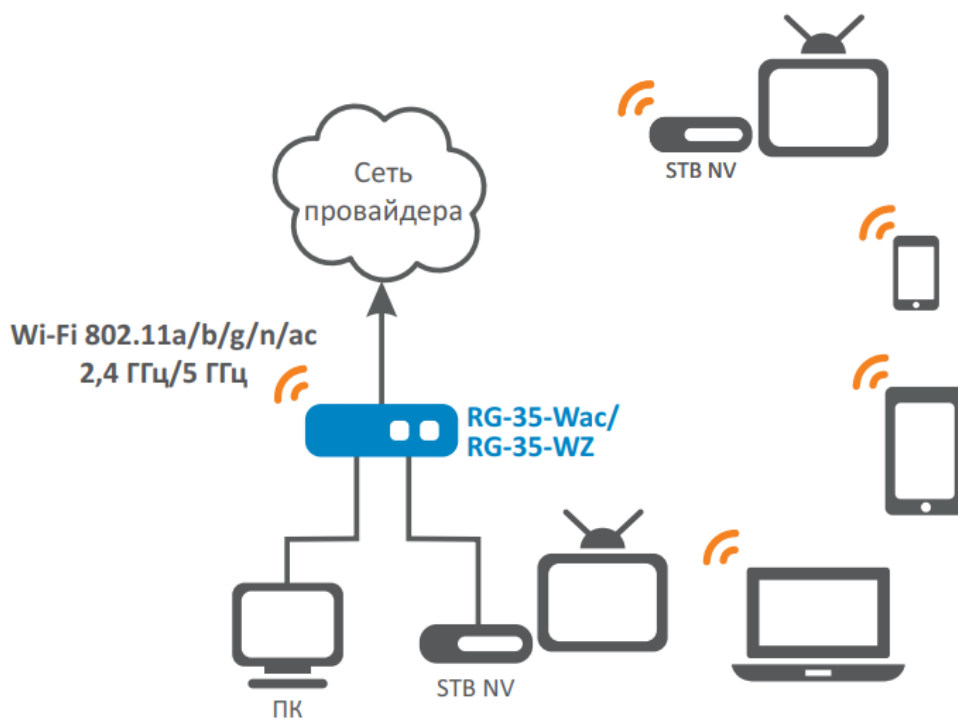
Рисунок 1 — Функциональная схема использования RG-35-WZ/Wac
