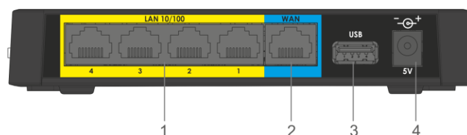
Рисунок 3 – Внешний вид задней панели RG-35-Wac/RG-35-WZ
