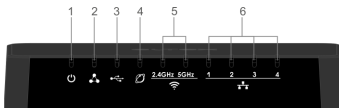
Рисунок 2 — Внешний вид передней панели RG-35-Wac/RG-35-WZ
