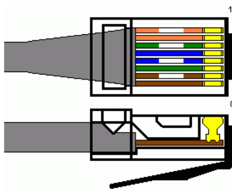
Рисунок 14 – Разъем RJ45
